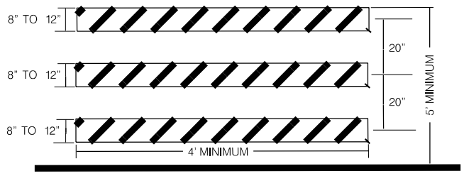
TYPE III BARRICADE
